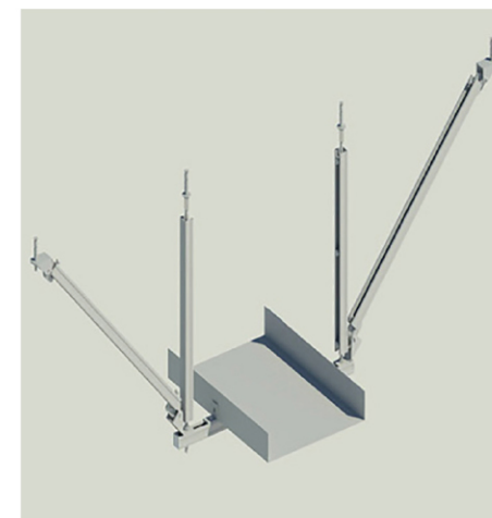
电缆桥架侧向支架 (T)
