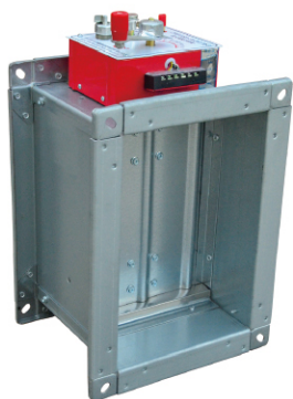
防火阀
