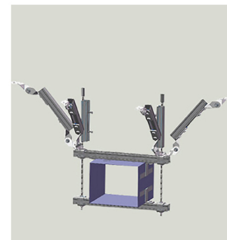
矩形风管纵向支架 (L)
