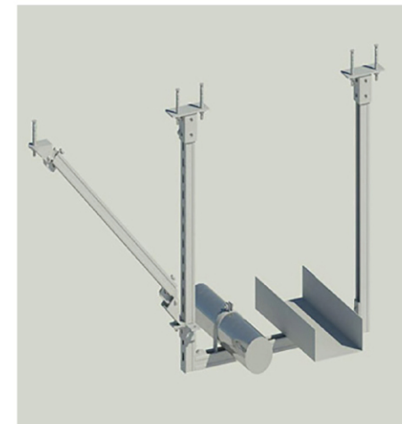
侧向抗震支架
